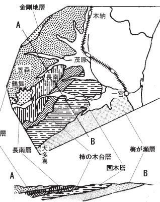
長南町周辺の地質 (原図・わがふるさと長南)
