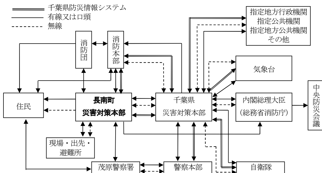
■災害通信系統図
