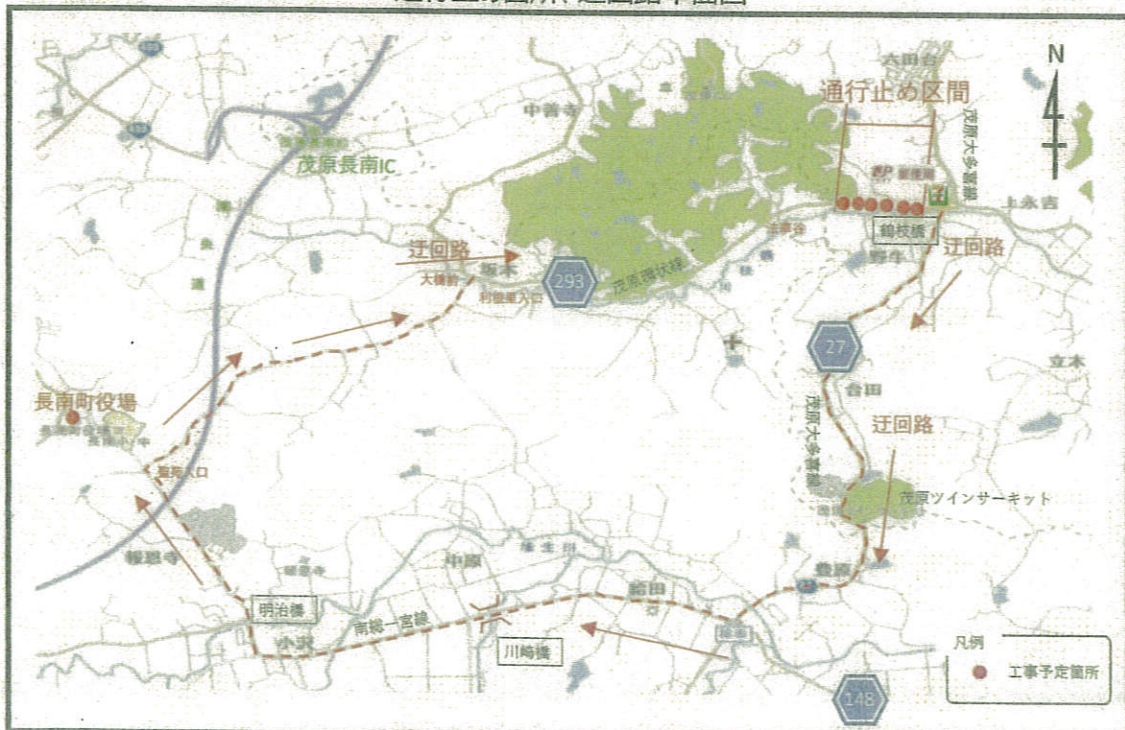
通行止め箇所、迂回路平面図
